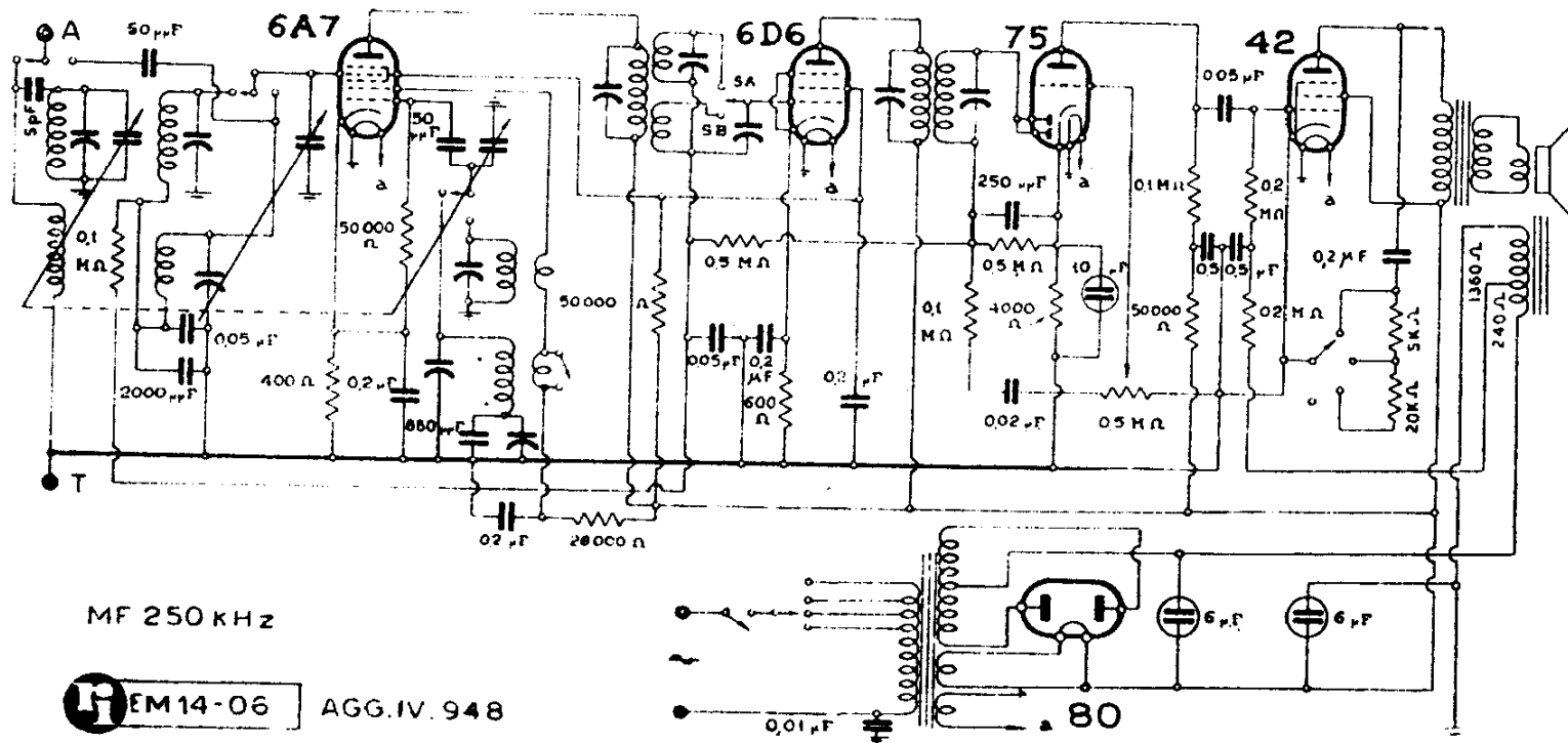
IRRADIO - MOD. « B 50 »
